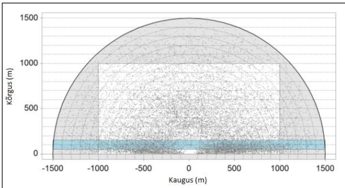
Joonis 10. Illustratsioon radarikontaktide kasutamisest. Hall poolring kujutab vertikaalse radari tööala raadiusega 1500 m, valge ristkülik maksimaalset ala mille kontakte kasutatakse lennu intensiivsuse arvutamiseks, sinine ristkülik ala mille kontakte kasutatakse kaugusest sõltuva avastatavustõenäosuse modelleerimiseks. Radari lähiümbruses (raadiusega ca 100 m) fikseeritud kontaktid praktiliselt puuduvad (Welcker 2019).
