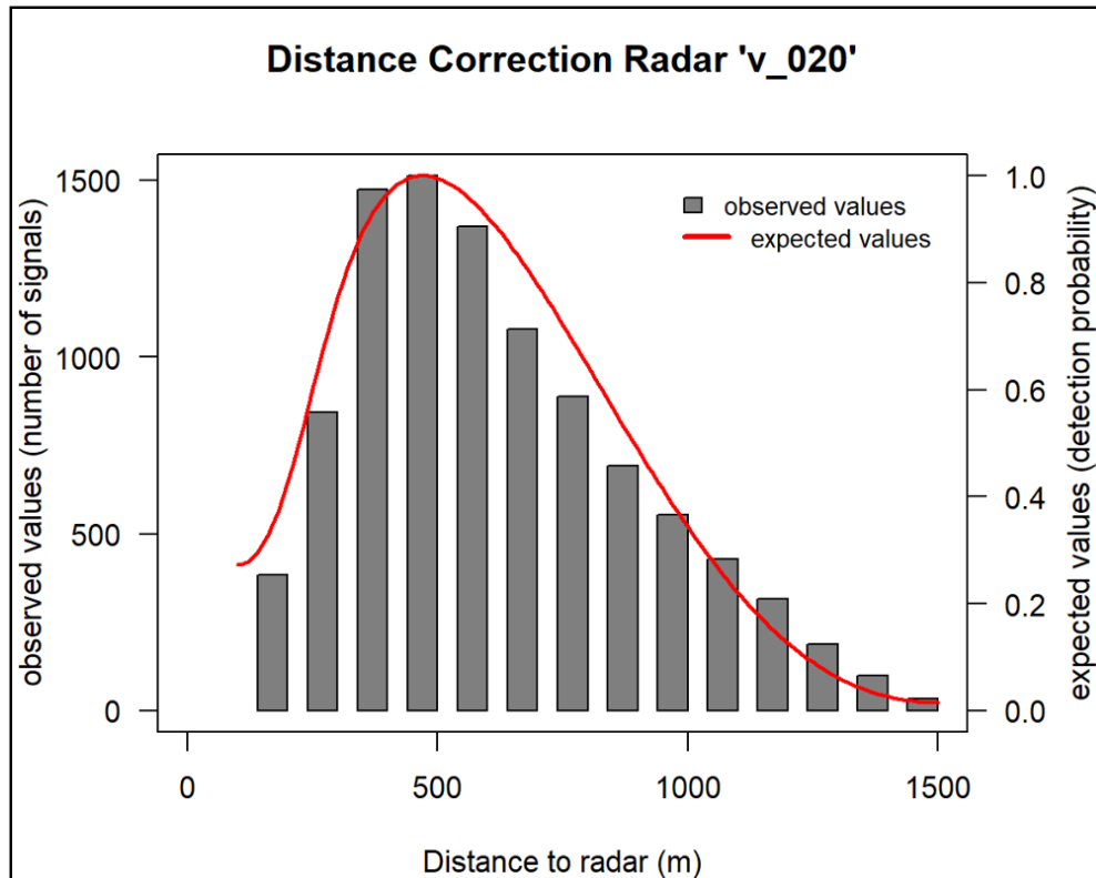
Joonis 11. Kaugusest sõltuv avastatavusfunktsioon laeval Arne Tiseliu kasutatud vertikaalse radari jaoks (horisontaalteljel kaugus radarist, meetrit; vertikaalteljel vasakul vaadeldud signaalide arv, vertikaalteljel paremal avastamise tõenäosus)
